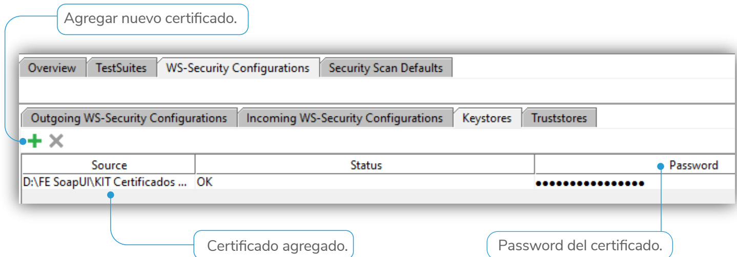
Ilustración 3. Configuración keystore
